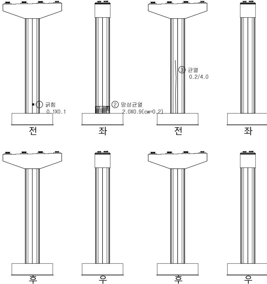
- 교각P1 -
