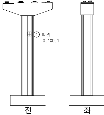
- 교각P4 -
