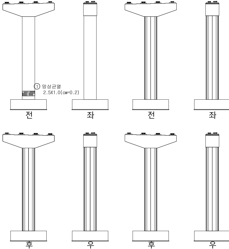
- 교각P5 -
